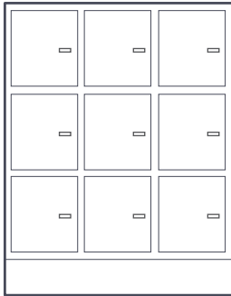
SF9/12 1228X910X372
