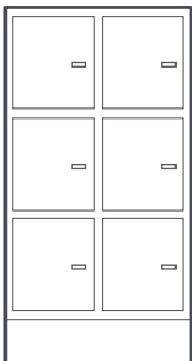
SF6/12 1228X613X372
