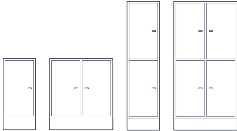
PDF4/9 876X410X580 PDF8/9 876X800X580 PDF4/15 1580X410X580 PDF8/15 1580X800X580
